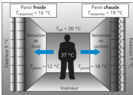
Figure 1 Température ressentie
