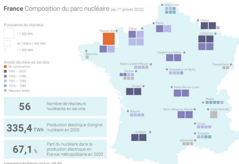
France Composition du parc nucléaire (au 1 er janvier 2022)
