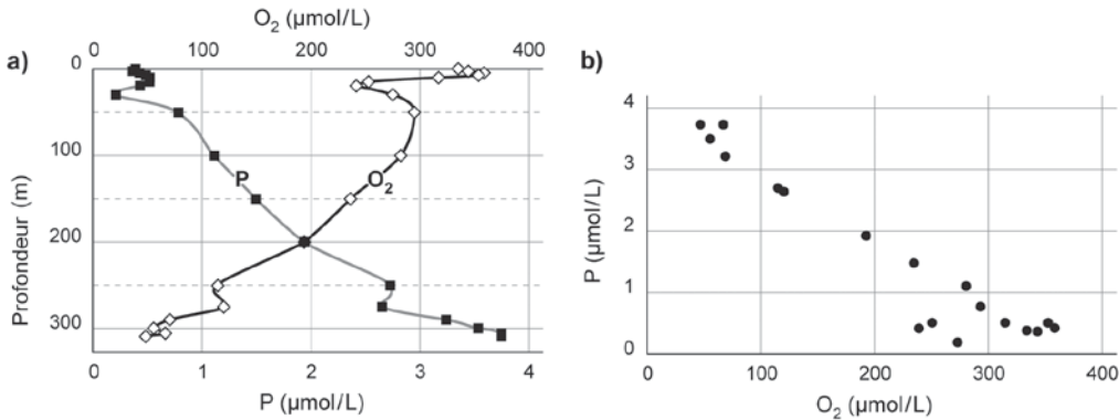
Figure 1.5 Concentrations en phosphate et oxygène dans le Lac Léman en été : a) en fonction de la profondeur ; b) relation entre P et O 2 .
