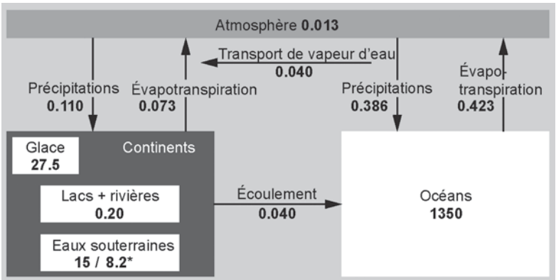
Figure 1.2 Cycle global de l'eau (réservoirs, volumes exprimés en 10^{15} \text{ m}^3 = 10^6 \text{ km}^3 ; flux d'eau en 10^{15} \text{ m}^3 \text{ an}^{-1} ).
