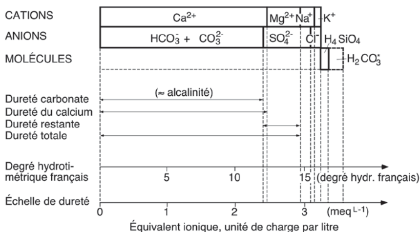
Figure 1.6 Composition des eaux européennes moyennes et leur échelle de dureté.
