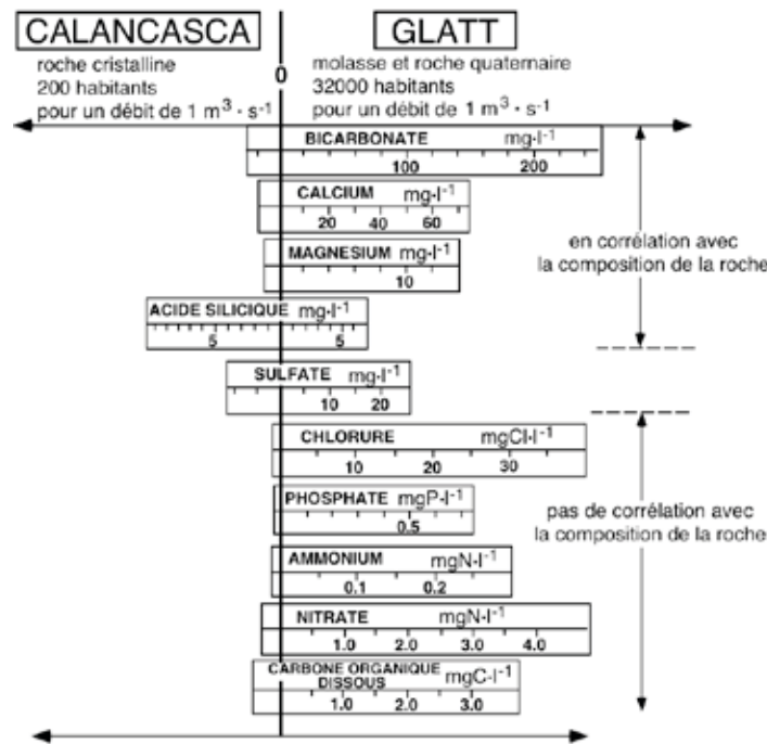
Figure 1.7 Comparaison entre la composition chimique du ruisseau Calancasca (sud de la Suisse), qui s'écoule au travers de roches cristallines, avec celle de la Glatt (plateau suisse), pour lequel les apports en CaCO 3(s) (calcite) sont importants. La Glatt subit aussi l'influence des apports de sels et de nutriments liée aux activités humaines.
