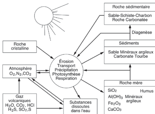
Figure 1.1 Interactions entre le cycle des roches et celui des eaux.
