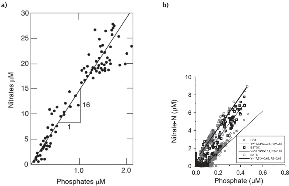
Figure 1.4 Corrélation stœchiométrique entre la concentration des nitrates et des phosphates (µM).
