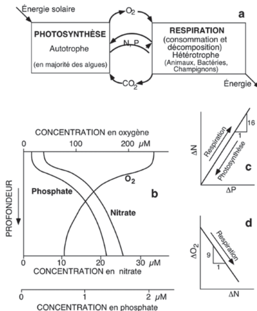
Figure 1.3 Un écosystème en équilibre est caractérisé par des conditions stables entre P (Vitesse de production par photosynthèse de la biomasse) et R (Vitesse de minéralisation par respiration de la matière organique).
