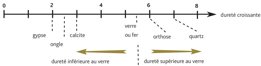
7 Échelle de dureté relative de Mohs
