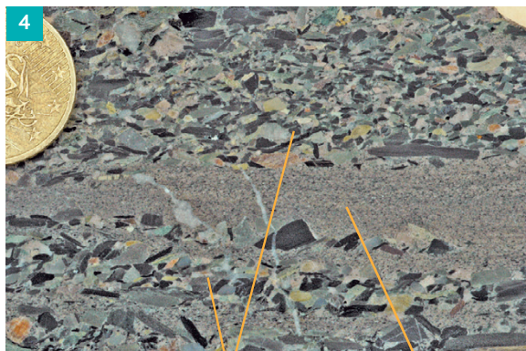
Texture litée d'une brèche
