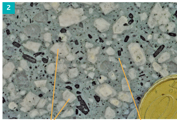
Texture microlitique d'une rhyolite
