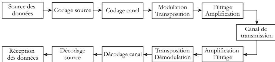
Figure 1.2 – Éléments fondamentaux d'une chaîne de transmission numérique
