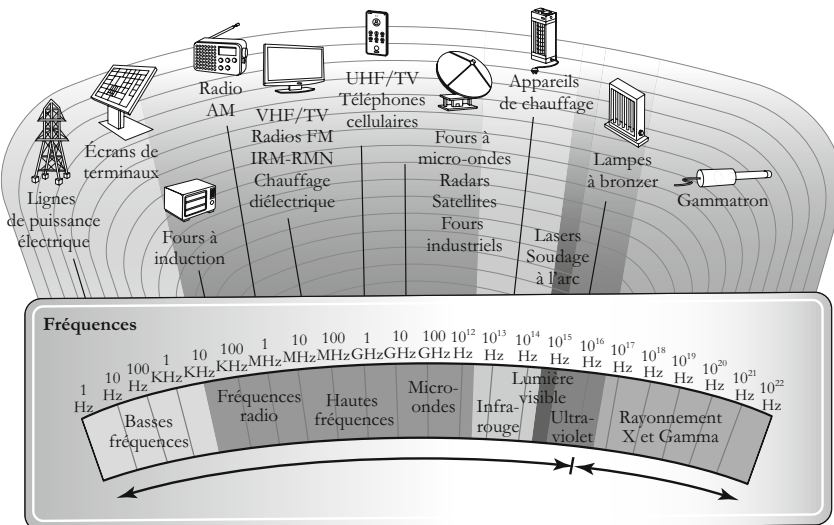
Figure 1.4 – Spectre des ondes électromagnétiques
