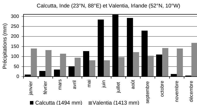
Figure A.1 – Comparaison de deux régimes pluviométriques ayant le même cumul annuel de précipitations.
