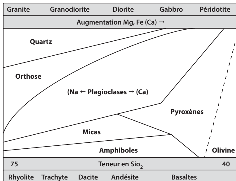
Figure 1.5 – Composition des principales roches éruptives (remarque : les roches riches en silice, mais dépourvues de quartz, syénite, ne figurent pas sur ce tableau).
