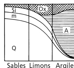
Figure 1.4 – Composition moyenne des fractions granulométriques (d'après BLUM et SCHRÖDER, 1992).
