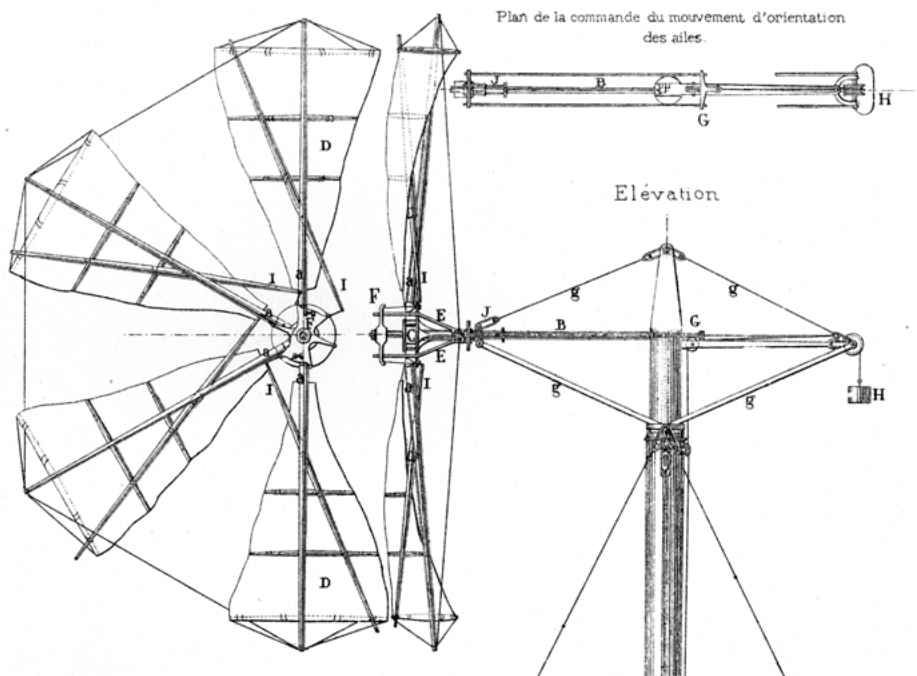
Figure 1.1 – Schéma de principe du moulin décrit par A. Durand en 1836 (collection M. Rapin)
