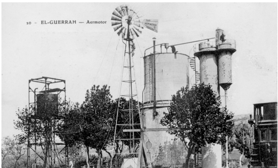
Figure 1.5 – Éolienne Aermotor en Algérie, début xx e siècle
