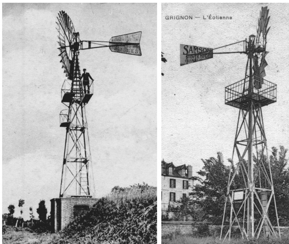
Figure 1.6 – Éoliennes Bompard Steel Star à Caumont-L'Éventé et Pilter Samson à Grignon (collection M. Rapin)
