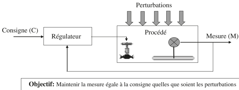
Figure 1.3 – Objectif de la régulation
