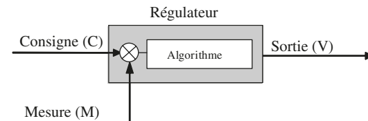
Figure 1.4 – Schéma de principe d'un régulateur
