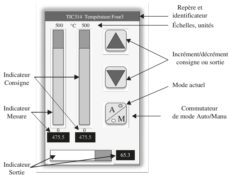
Figure 1.6 – Synthèse d'une face avant
