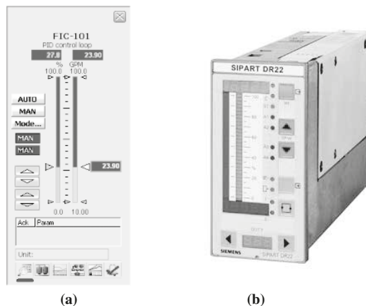
Figure 1.5 – Exemples de face avant. a : face avant régulateur, système Emerson Delta V ; b : face avant régulateur, Siemens Sipart DR22
