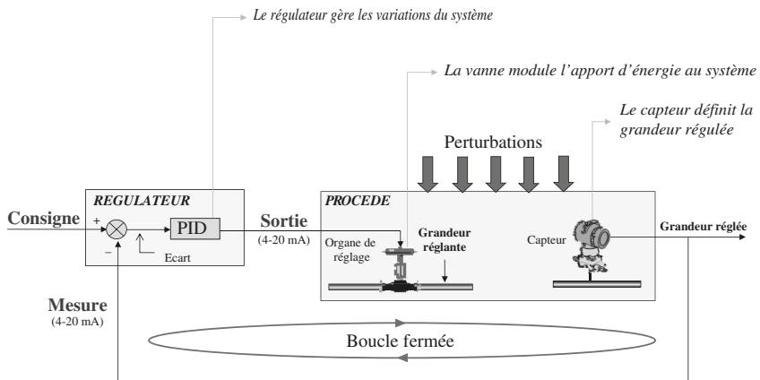
Figure 1.2 – Schéma de principe d'une boucle simple
