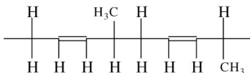
Séquence de deux unités monomères successives (diade) de cis-1,4-polypentadiène, présentant des chiralités opposées et des configurations géométriques identiques.
