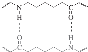
Figure 2.3 - Liaisons hydrogène dans le polycaprolactame (PA-6).
