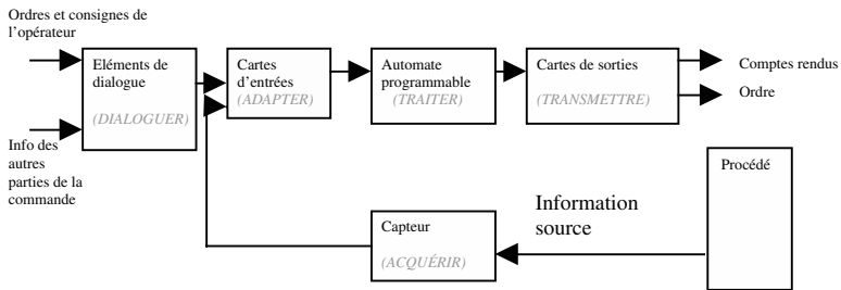
Figure 1.6 Chaîne d'information.
