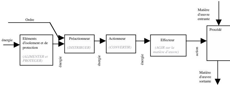
Figure 1.5 Chaîne d'action.
