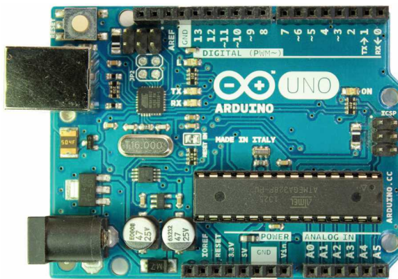
Figure 1.3 La carte Arduino Uno
