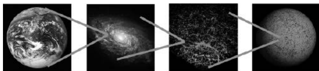
Figure 2.2 Chaque fois que nous sommes parvenus à prendre de la distance, nous avons découvert que tout ce que nous savions n'était qu'une partie d'un ensemble plus vaste : notre pays est situé sur une planète (à gauche), qui appartient à un système solaire, qui compose une galaxie (milieu gauche), qui dessine le motif cosmique d'un amas de galaxies (milieu droite), qui fait partie de notre Univers observable (à droite), qui pourrait contribuer à un ou plusieurs niveaux d'univers parallèles.
