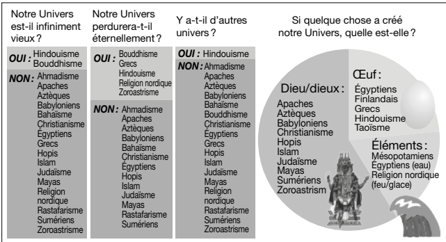
Figure 1.2 Plusieurs des questions cosmologiques qui nous tarauderont tout au long de ce livre ont fasciné les penseurs à travers les siècles, mais aucun consensus global n'a pu émerger. La classification reproduite ci-dessus se fonde sur une présentation donnée par un étudiant du MIT, David Hernandez, pour mon cours de cosmologie. De telles taxinomies sont beaucoup trop simplistes et doivent être prises avec des pincettes : de nombreuses religions exhibent plusieurs branches et interprétations, et certaines d'entre elles tombent dans plusieurs catégories. Par exemple, l'hindouisme fait appel aux trois sources de création mentionnées : selon l'une des légendes, le dieu créateur Brahma (représenté) et notre Univers ont tous deux émergé d'un œuf qui lui-même proviendrait de l'eau.
