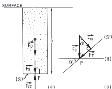
Figure 2.3 – Force de pesanteur \mathbf{F}_p agissant sur une colode roche et force de surface \mathbf{F}_s agissant sur sa base horizontale (S).
