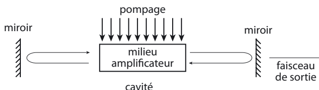
Figure 2 – Représentation schématique d'un oscillateur du domaine optique.
