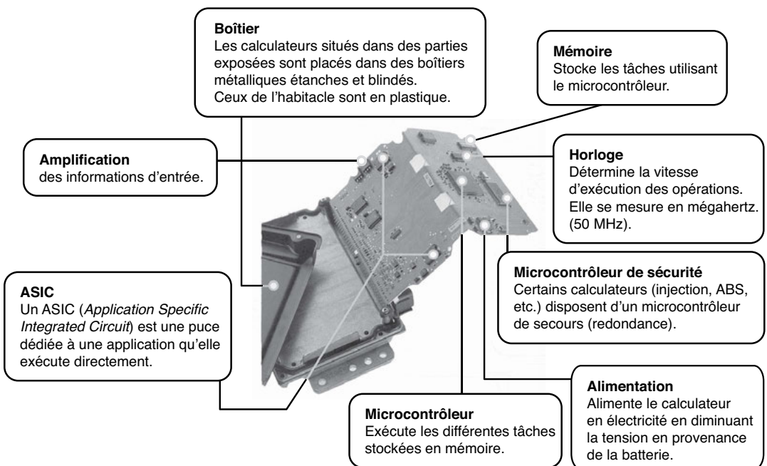
Figure 1.12 Matériel dédié utilisé pour implémenter une application de contrôle-commande du domaine de l'automobile.
