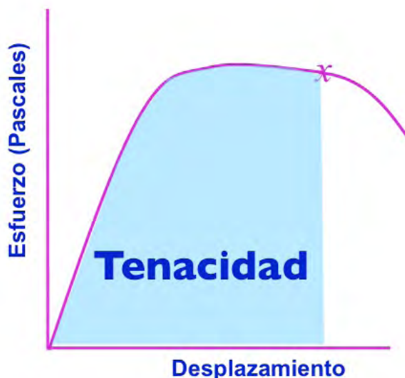
Figura 1.3. Curva esfuerzo-deformidad.
