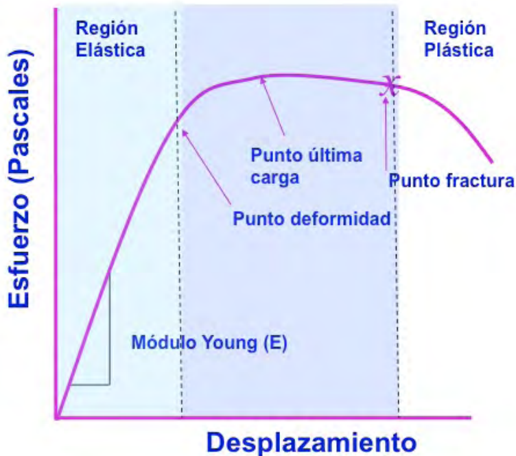
Figura 1.2. Curva carga-desplazamiento.
