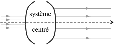
Figure 2.9 – Système afocal.
