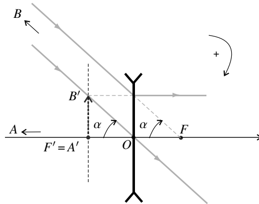
Figure 2.25 – L'objet réel est à l'infini. L'image est virtuelle, droite.
