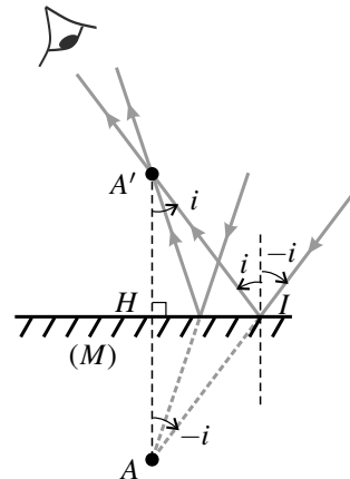
Figure 2.2 – Image d'un point objet virtuel par un miroir plan.
