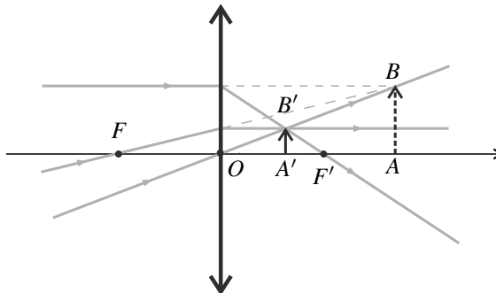
Figure 2.20 – L'objet virtuel est situé après le centre. L'image est réelle, droite, rétrécie.
