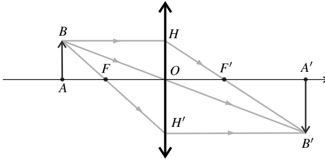
Figure 2.18 – L'objet est réel situé avant le foyer objet. L'image est réelle, renversée, agrandie.
