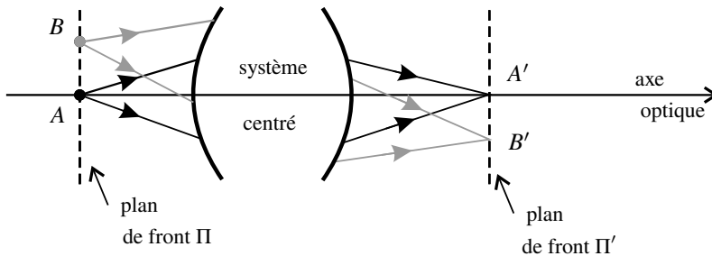
Figure 2.4 – Stigmatisme et aplanétisme dans les conditions de Gauss.
