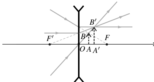
Figure 2.23 – L'objet virtuel situé entre le centre et le foyer objet. L'image est réelle, droite, agrandie.
