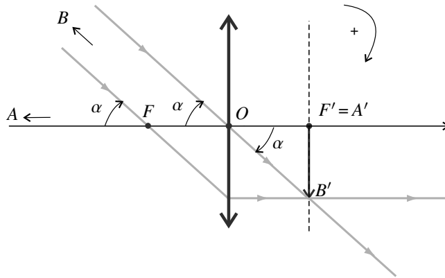
Figure 2.21 – L'objet réel est à l'infini. L'image, est réelle, renversée.
