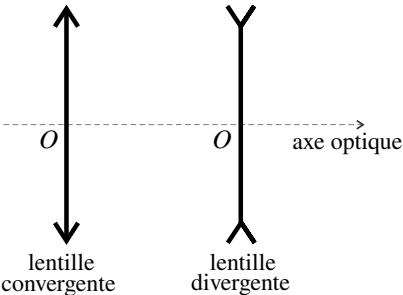
Figure 2.13 – Symbole des lentilles minces.
