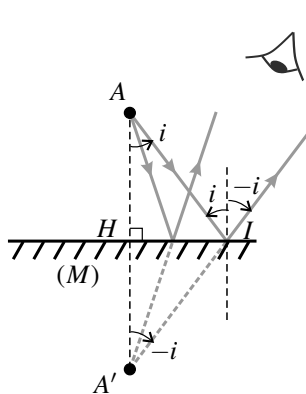
Figure 2.1 – Image d'un point objet réel par un miroir plan.
